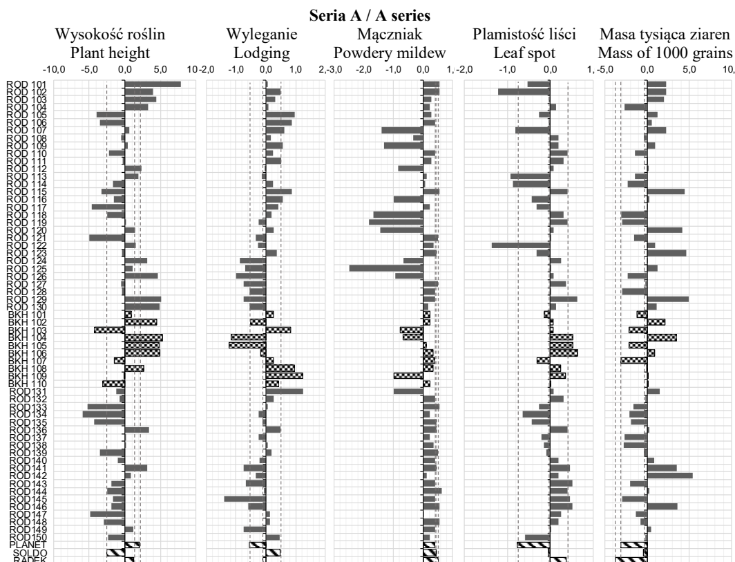
Rys. 3 a. Zestawienie wartości BWLUE dla wysokości roślin, wylegania, mączniaka, plamistości liści oraz masy tysiąca ziaren rodów i odmian badanych w zespołowych doświadczeniach hodowlanych z jęczmieniem jarym w roku 2016. Jednolite szare słupki oznaczają wartości efektu BWLUE dla plonów rodów pochodzących z innych hodowli niż HR Smolice, rody z HR Smolice oznaczono kratkowanymi słupkami, a odmiany wzorcowe słupkami prążkowanymi. Linie przerywane oznaczają poziom efektów dla odmian wzorcowych
